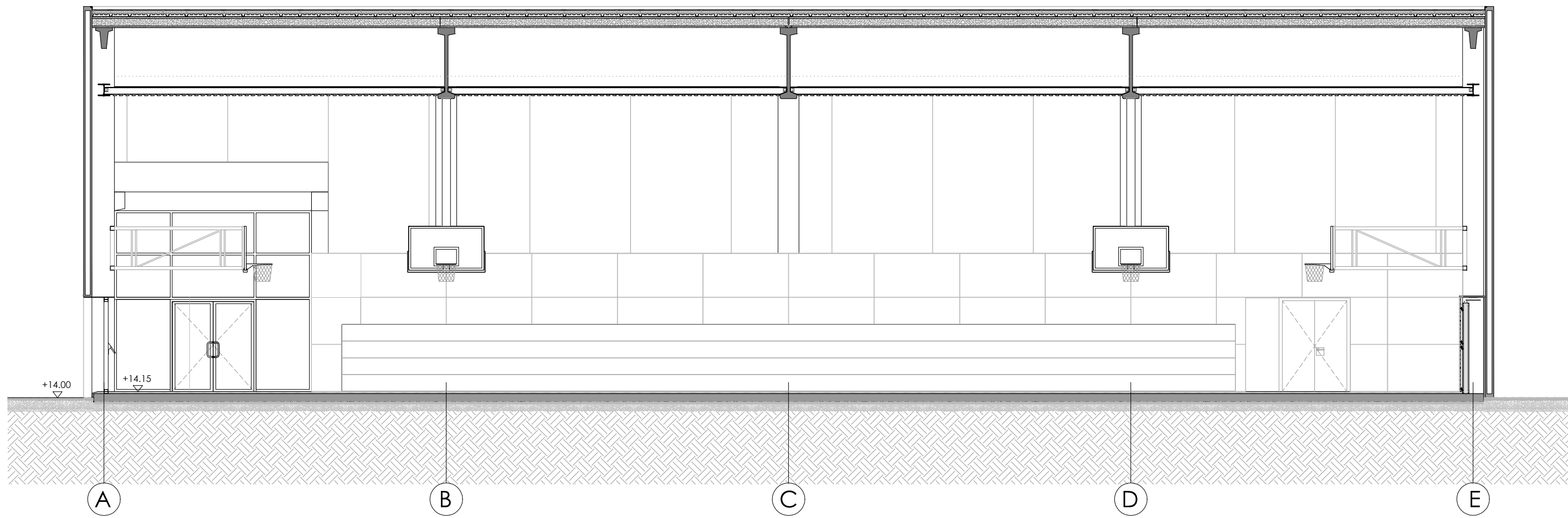
SECCIÓ TRANSVERSAL PISTA POLIESPORTIVA: T-02
