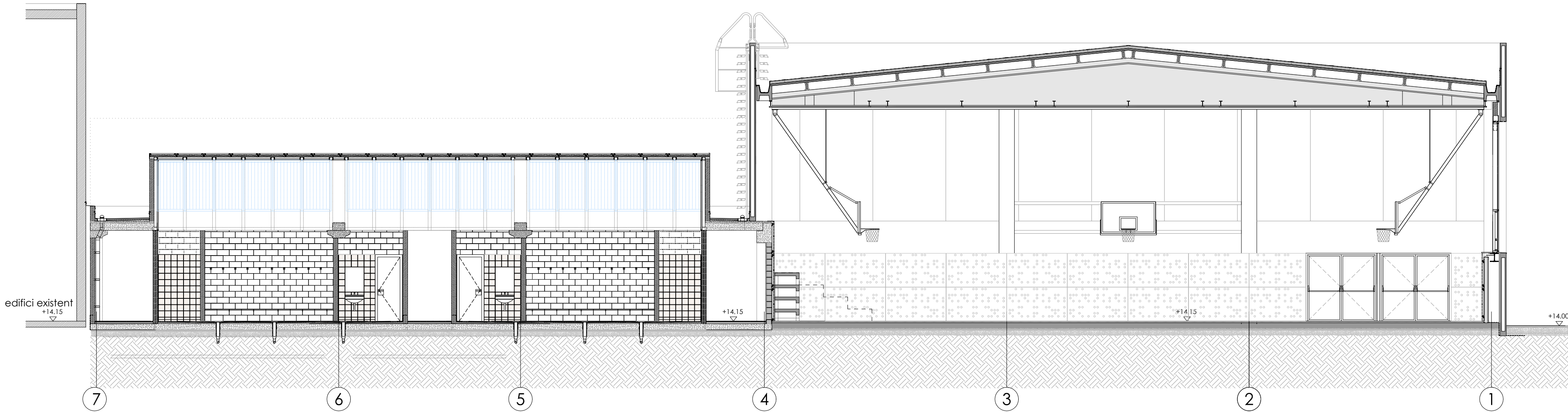
SECCIÓ LONGITUDINAL VESTIDORS-PISTA : L-01
