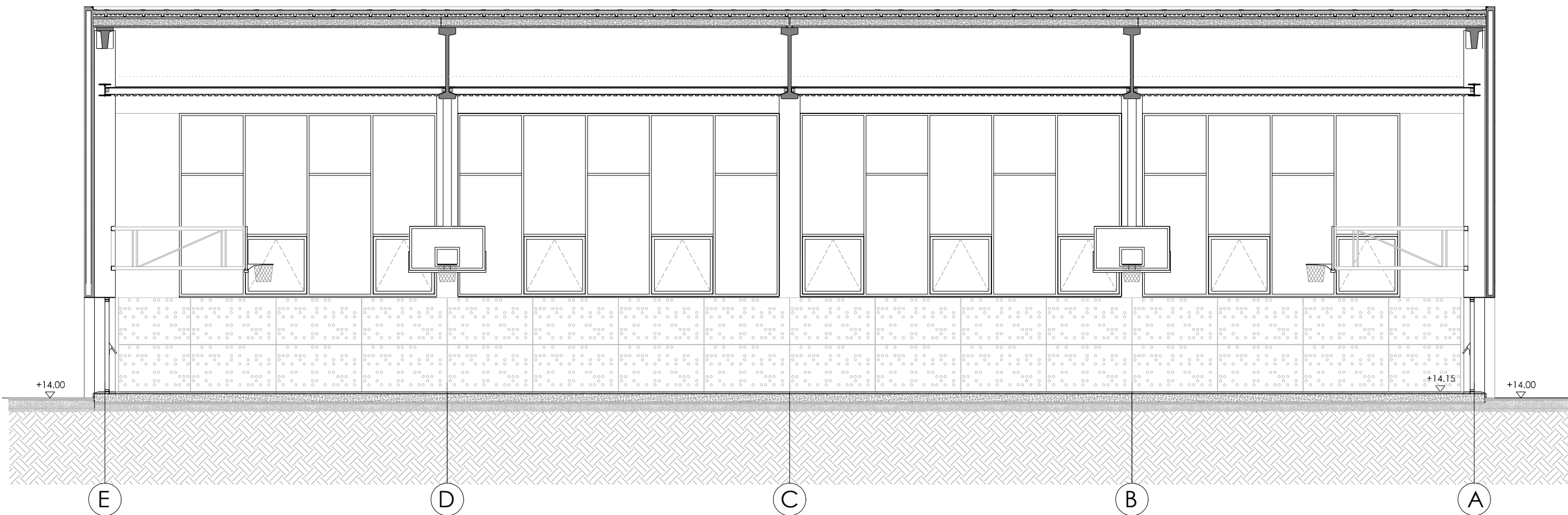
SECCIÓ TRANSVERSAL PISTA POLIESPORTIVA: T-03
